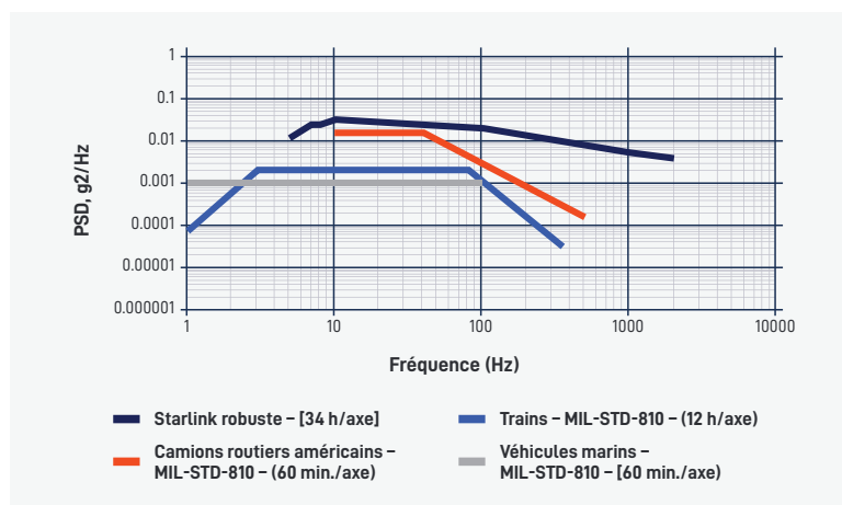
Schéma 1 : comparaison des profils de test de vibration d'utilisation courante – Axe vertical
