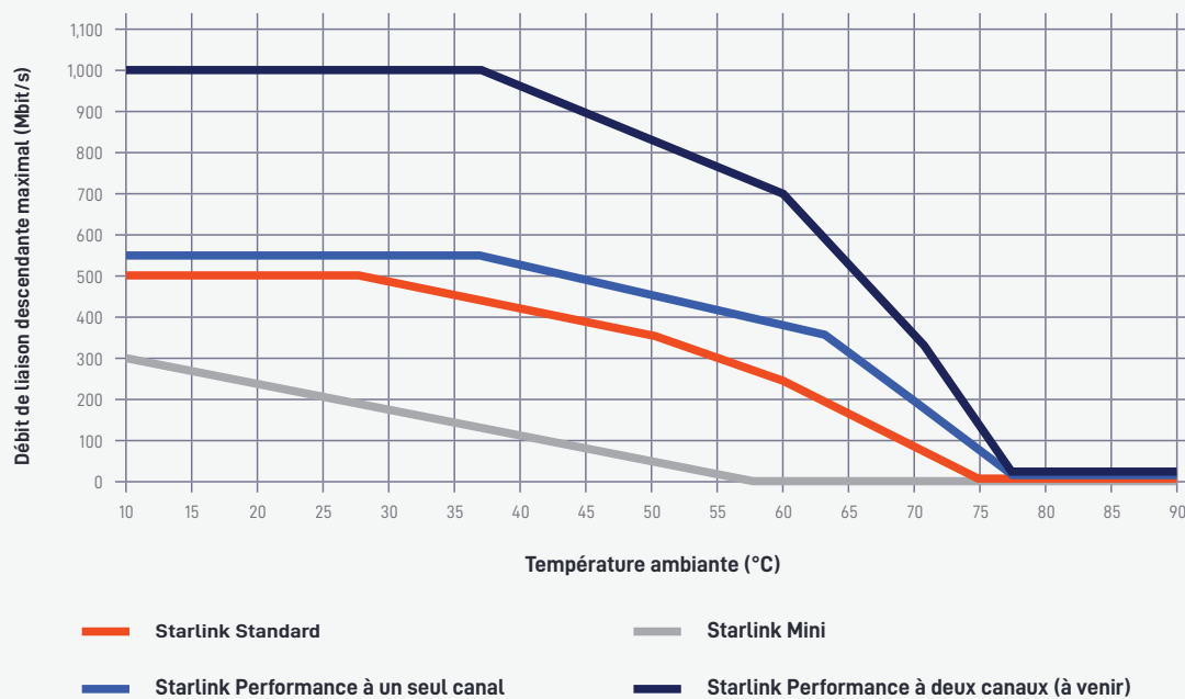
Schéma 2 : débit par rapport à la température ambiante avec charge solaire complète
